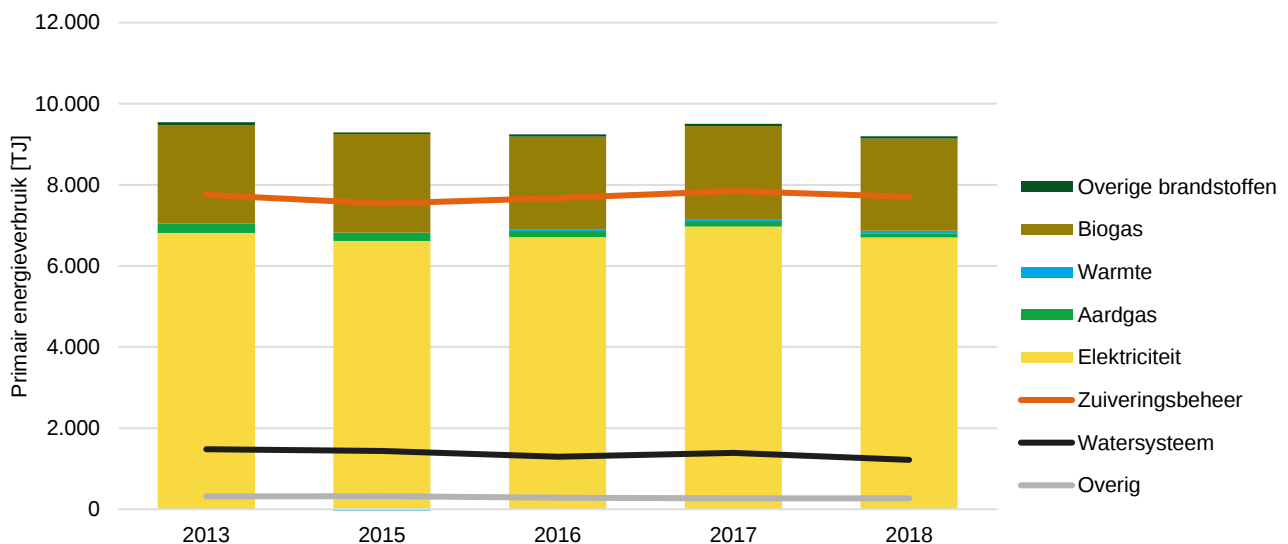
Figuur 10 Primair energieverbruik 2013-2018 per energiedrager en bedrijfsonderdeel
