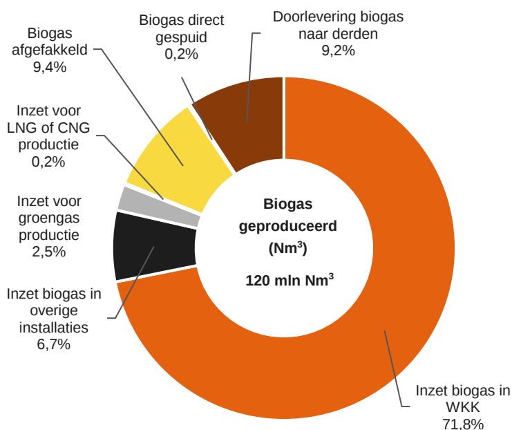
Figuur 8 Toepassing van de hoeveelheid (Nm³) geproduceerd biogas, inclusief spui (scope 1).
