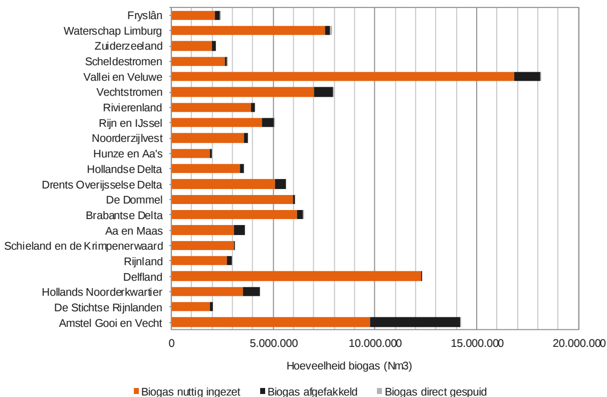
Figuur 21 Geproduceerd biogas en gebruikswijze voor alle waterschappen in 2018
