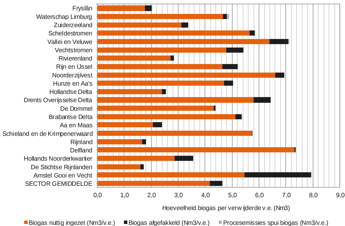
Figuur 22 Biogasproductie per verwijderde vervuilingseenheid voor alle waterschappen
