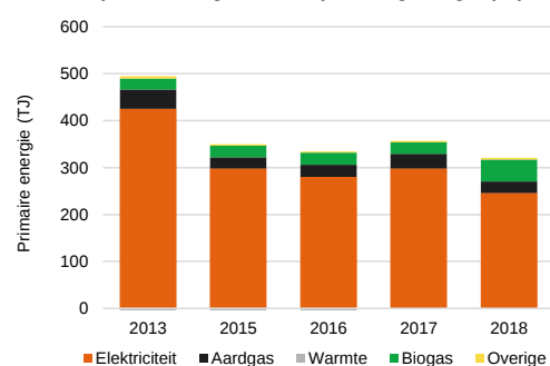
Trend primair energieverbruik per energiedrager (TJ)
