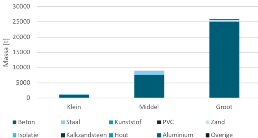
AFBEELDING 3.1 MATERIALISATIE REFERENTIE RWZI'S
