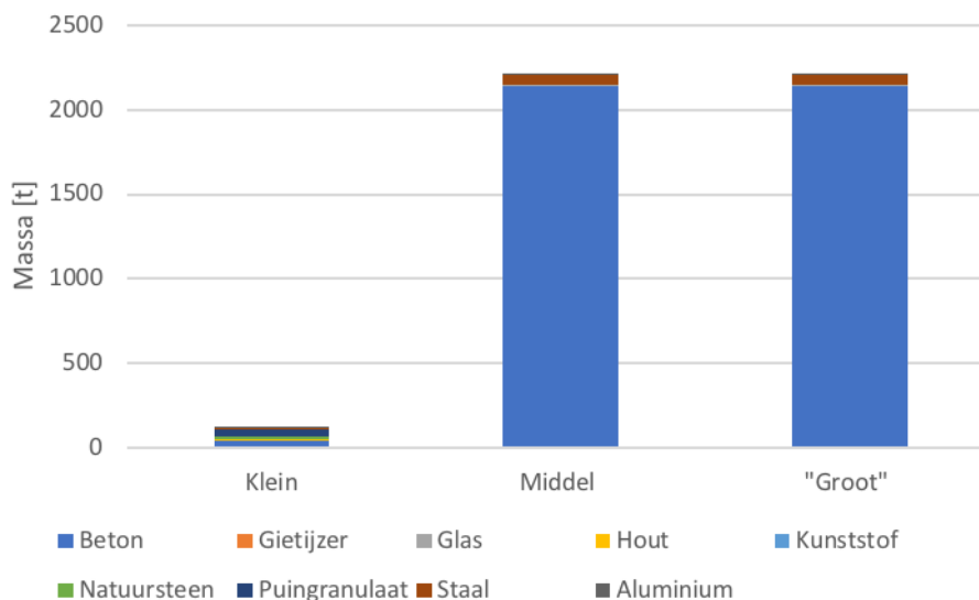
AFBEELDING 3.5 MATERIALISATIE REFERENTIE POLDERGEMALLEN
